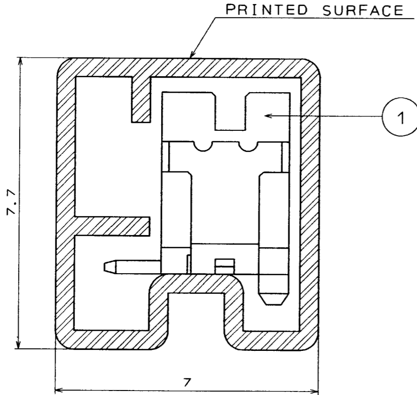
A-A SECTION (10:1)
