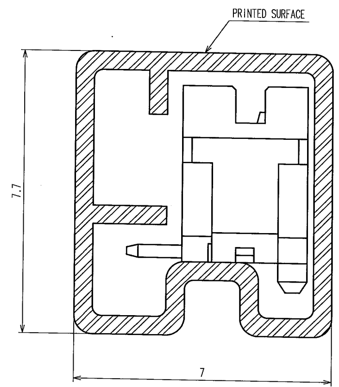
A-A SECTION (10:1)
