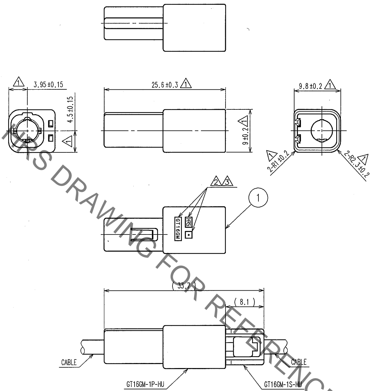
使用状態かん合図 MATED CONNECTORS
