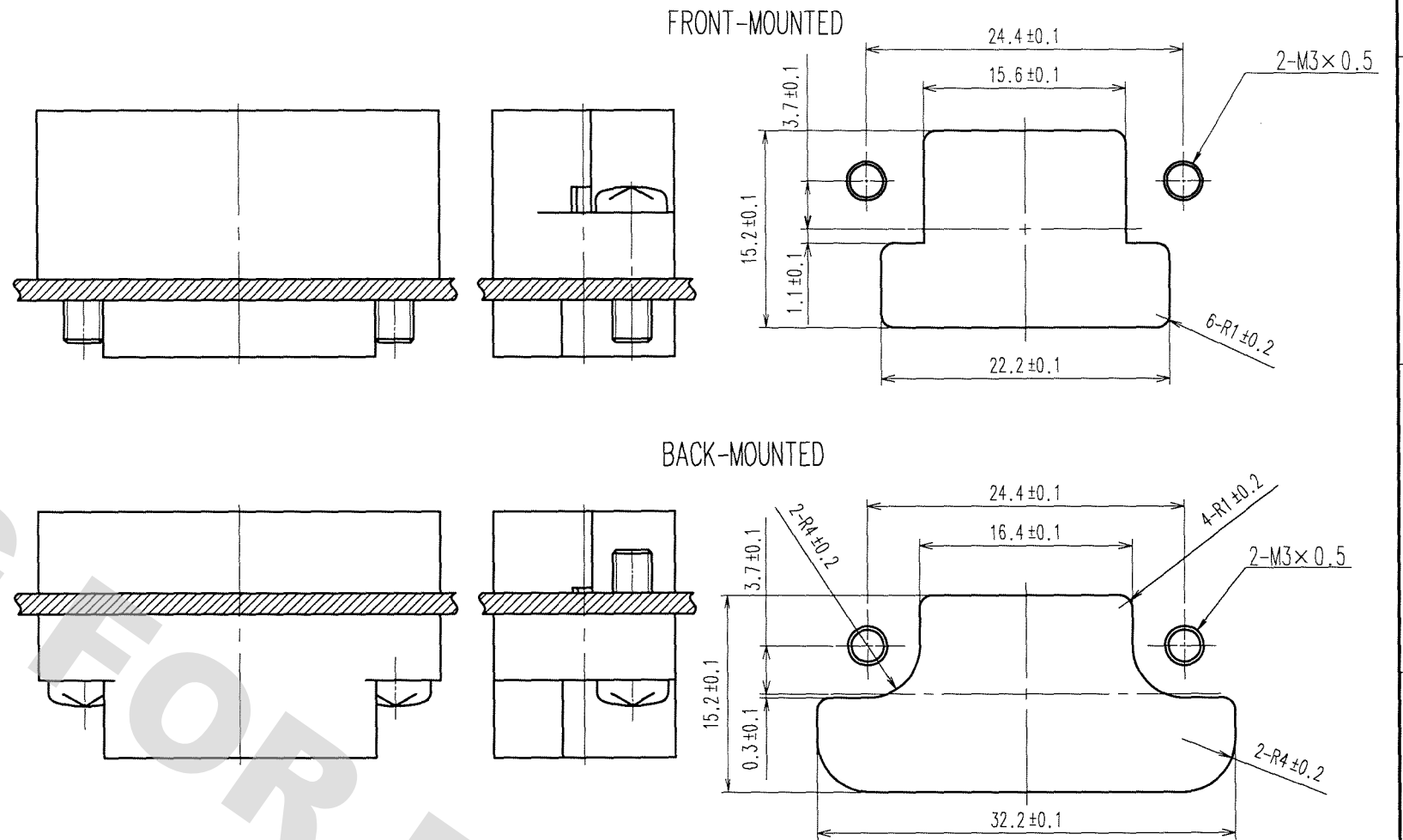
PANEL CUTOUT ( 2:1 )
