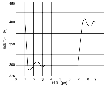
图8: 电压跟随器脉冲响应 (大信号)
