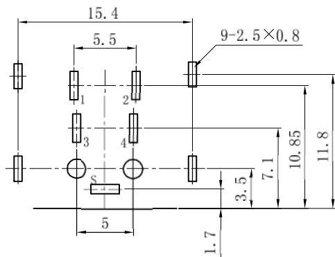
PCB板安装孔图
