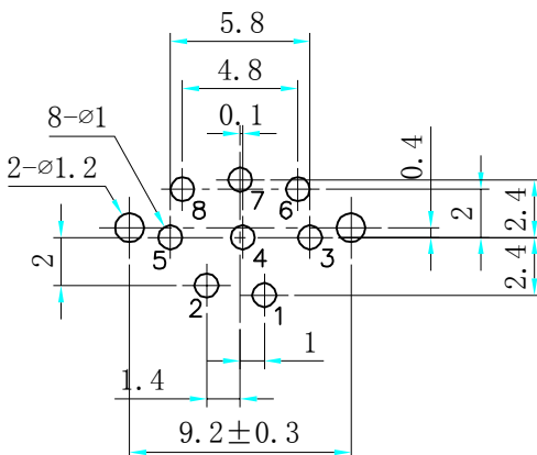
PCB板安装孔图
