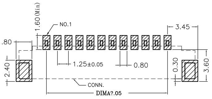
适用线路板 (PCB LAYOUT)
