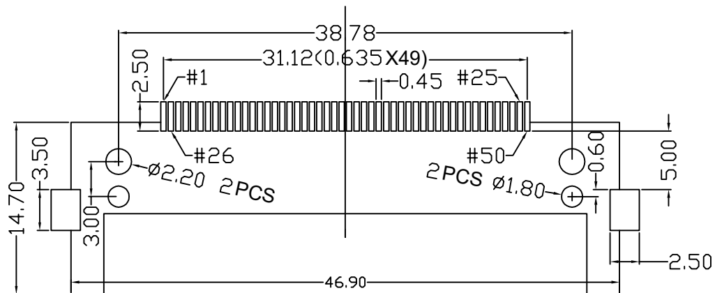
P.C.Board layout
