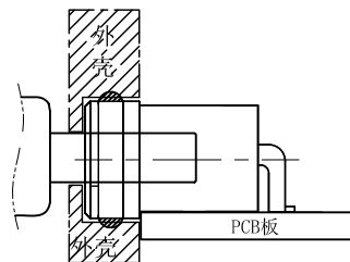
组装示意图
