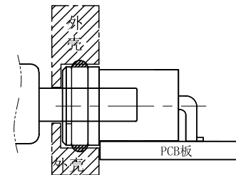
组装示意图
