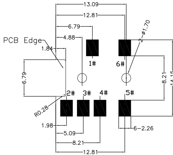
P.C.B LAYOUT
