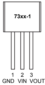
TO92
