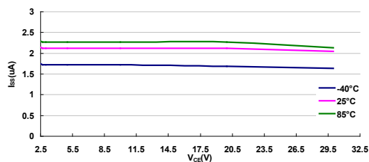
I_{SS} vs V_{CE} : HT7333-7 ( I_{OUT}=0mA )
