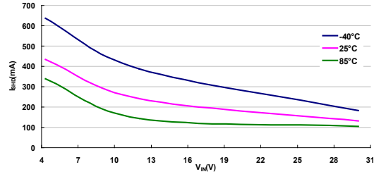
Iq VS VIN
