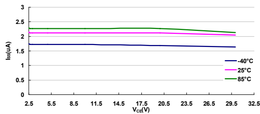
I_{SS} vs V_{CE} : HT7350-7 ( I_{OUT}=0mA )
