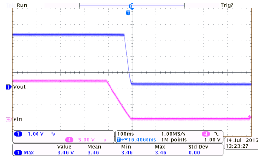
掉电响应： HT7333-1 ( I_{OUT}=0mA , T_{FALL}=100ms )
