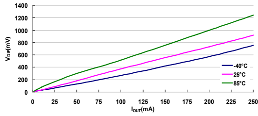
压差: HT7350-7
