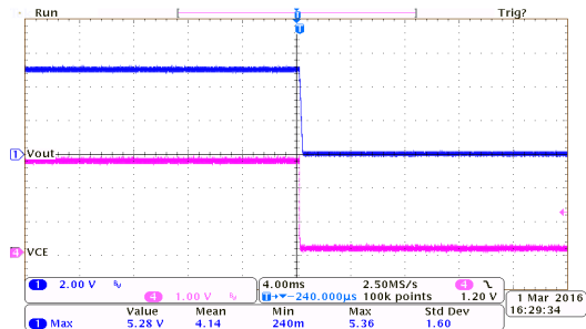
掉电响应:
