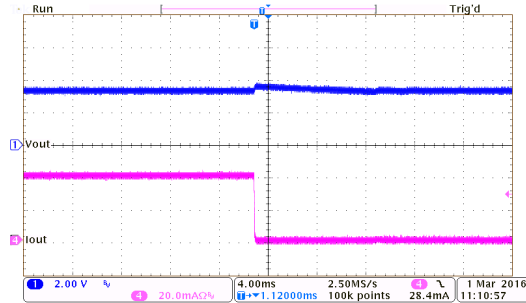
负载瞬态响应： HT7333-7 ( V_{IN}=5.3V , I_{OUT}=40mA to 0mA )
