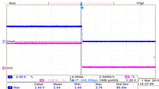
掉电响应:
