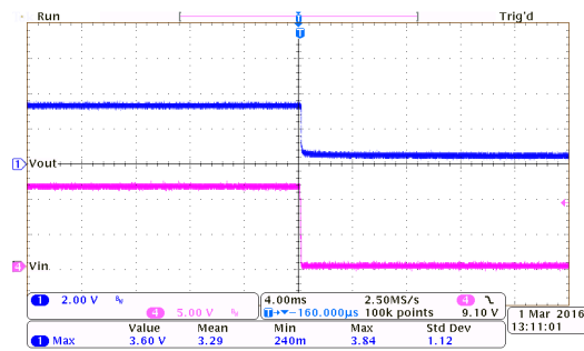
掉电响应:
