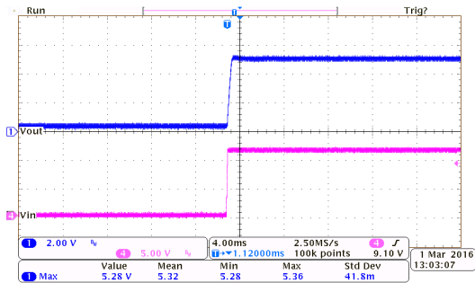
上电响应:
