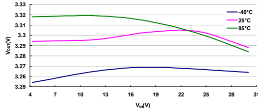
线性调整率: HT7333-7 ( I_{OUT}=10mA )
