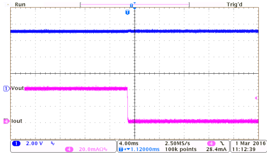
负载瞬态响应： HT7350-7 ( V_{IN}=7.0V , I_{OUT}=40mA to 0mA )
