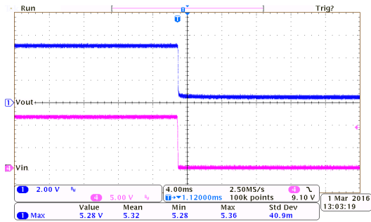
掉电响应:
