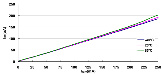
I_{SS} vs I_{OUT} : HT7333-7 ( V_{IN}=5.3V )
