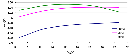
线性调整率: HT7350-7 ( I_{OUT}=10mA )
