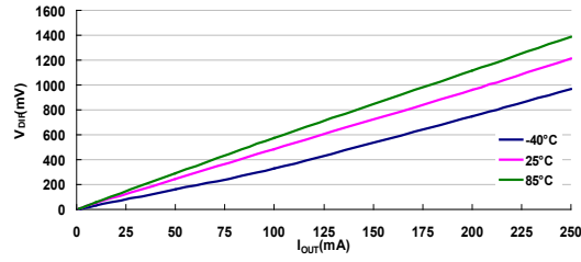
压差: HT7333-7
