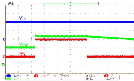
HT7733B Chip Enable/Disable
