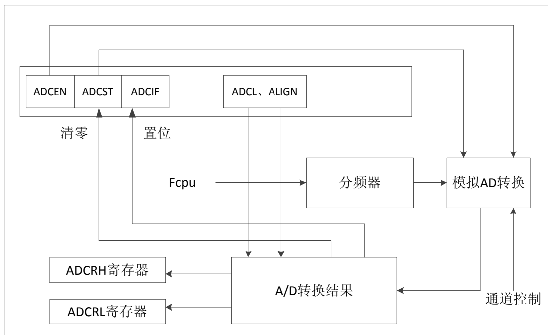
Figure 18-1 ADC 功能框图
