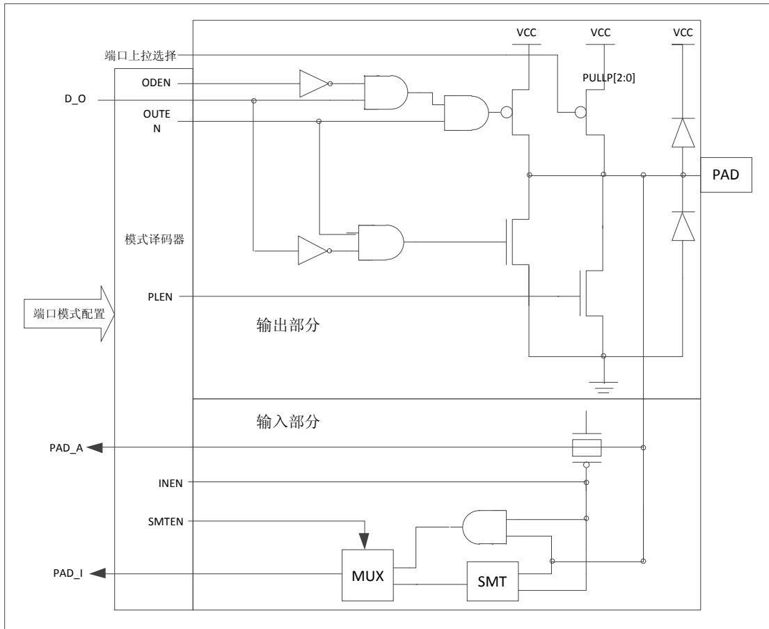
Figure 7-1 I/O 功能框图
