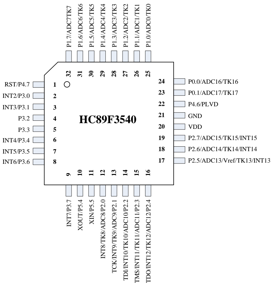
Figure 1-2 LQFP32/QFN32 引脚配置图
