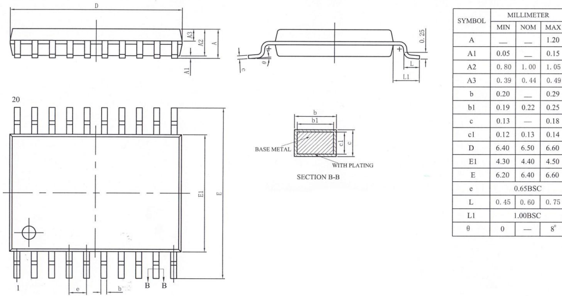
Figure 24-5 TSSOP20 封装尺寸
