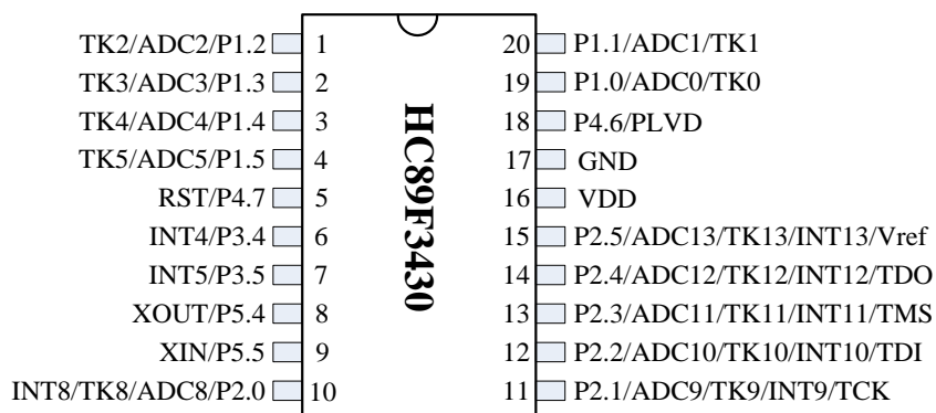
Figure 1-3 DIP20/SOP20/TSSOP20 引脚配置图
