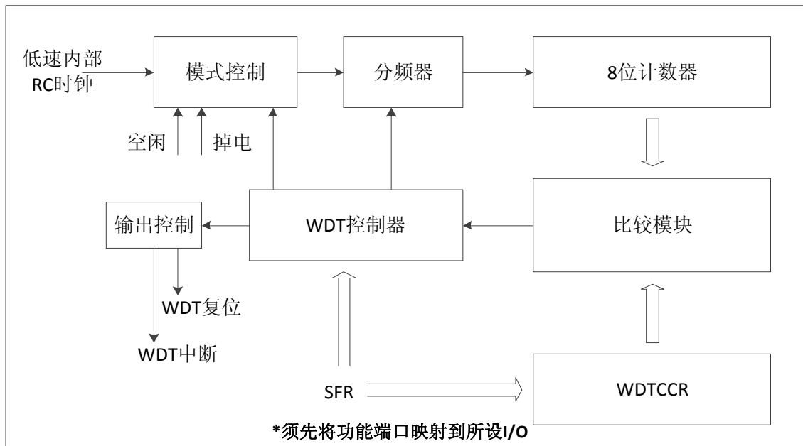
Figure 13-1 WDT 功能框图
