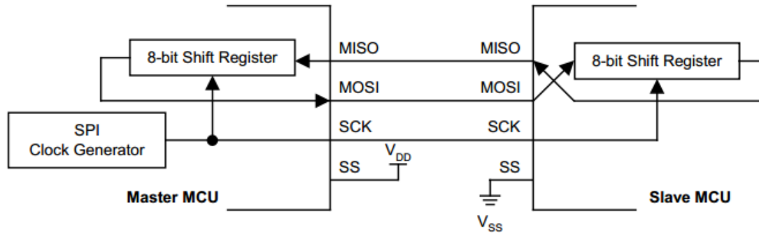
Figure 15-2 全双工主从互联图
