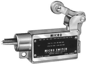
Right-hand actuator
