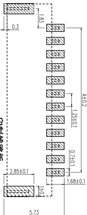
印制线路板
