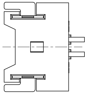
2~3 Pin结构外形(锁扣窗口)
