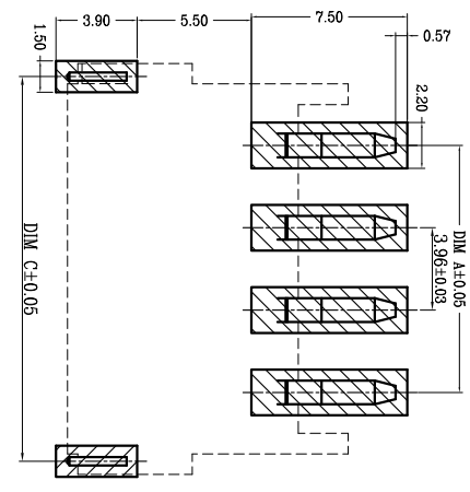
适用线路板(厚度: 0.8mm~1.6mm)
