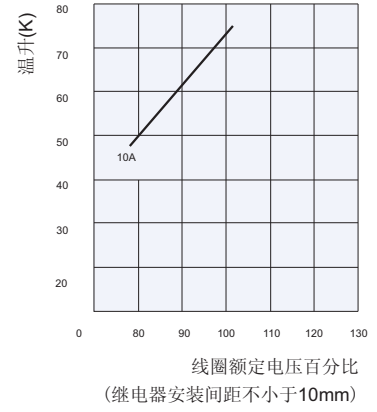
线圈温升
