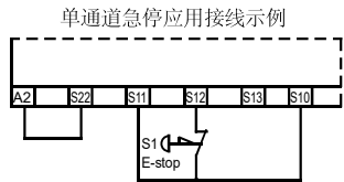
ESL急停监控功能典型示例
