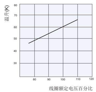
线圈温升
