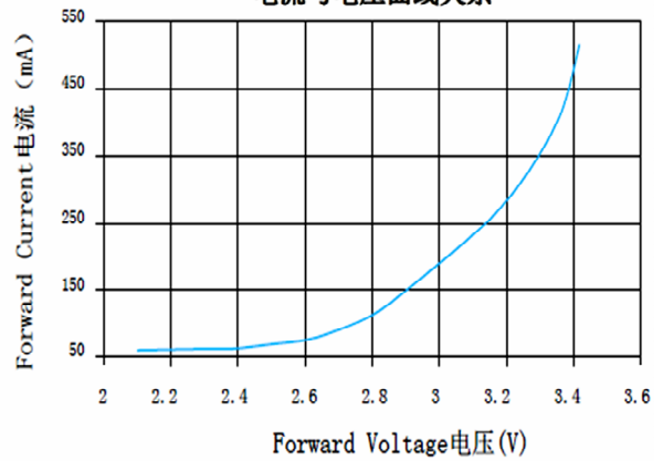
Forward Current vs. Forward Voltage 电流与电压曲线关系
