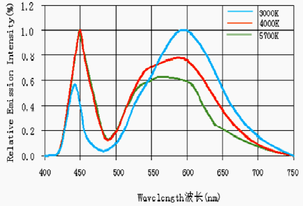
Spectrum Distribution 光谱分布图
