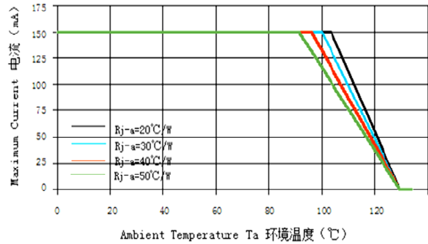
Thermal design 电流与环境温度曲线关系
