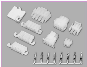
端子 TERMINAL(63080)
