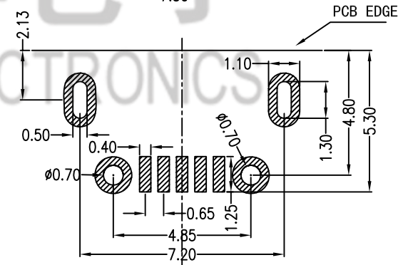
PCB 图仅作参考
