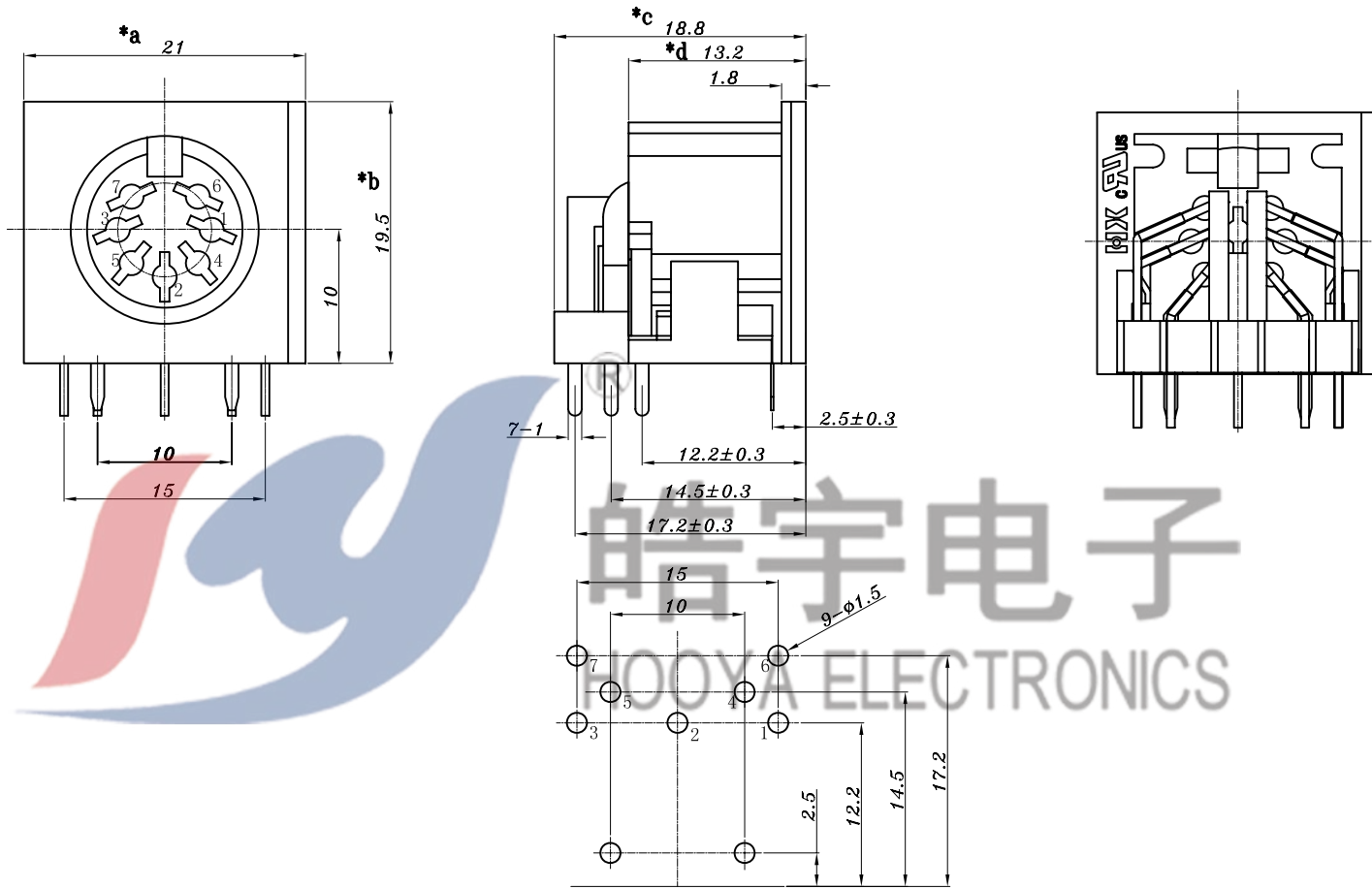
PCB板安装孔图
