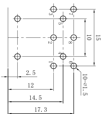
PCB板安装孔图
