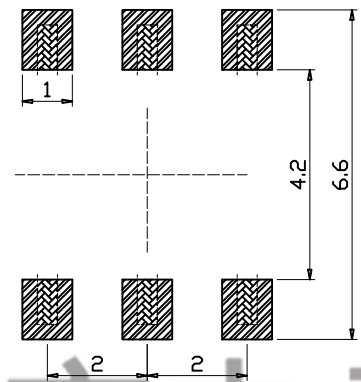
安装图 (PCB LAYOUT PLAN)
