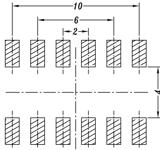
P.C.B LAYOUT
