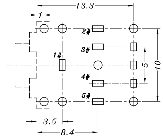
P.C.B LAYOUT
