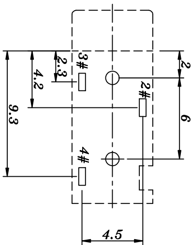
P.C.B LAYOUT
