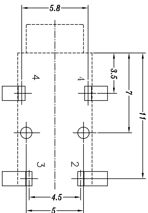
P.C.B LAYOUT
