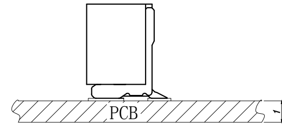
截面 A-A
