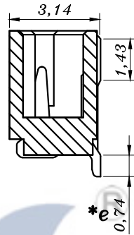
截面 A-A
