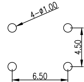
PCB. 焊接图
