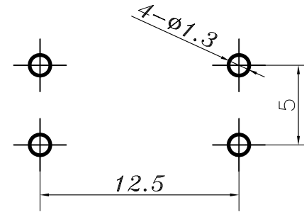
PCB. 焊接图
