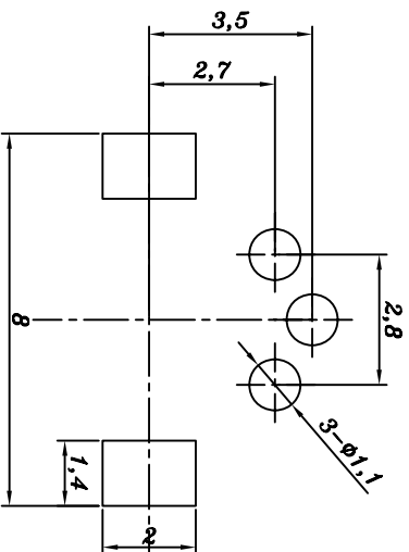
安装尺寸图
