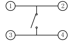
电路图
