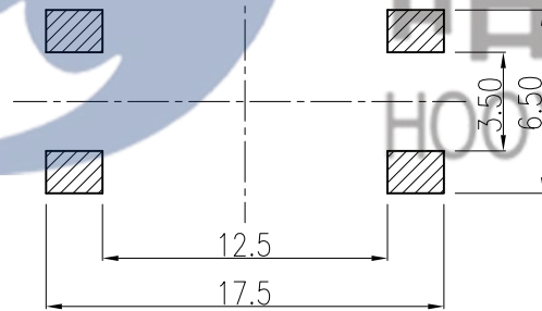
PCB. 焊接图
