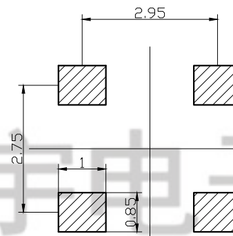
安装参考图
