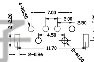
PCB板孔位
