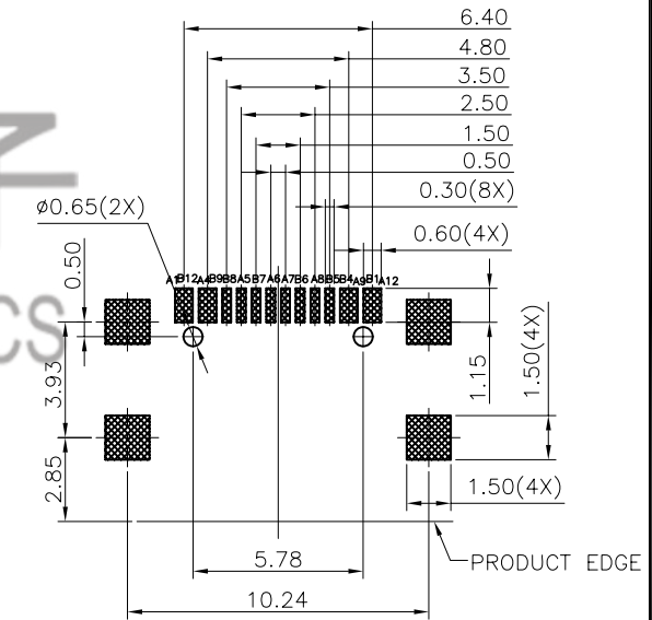
P.C.B LAYOUT
