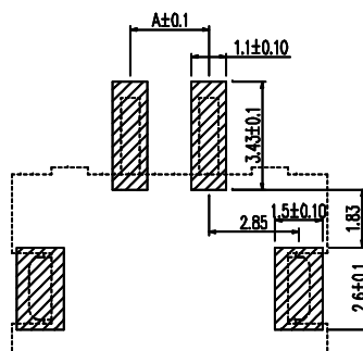
印制线路板
