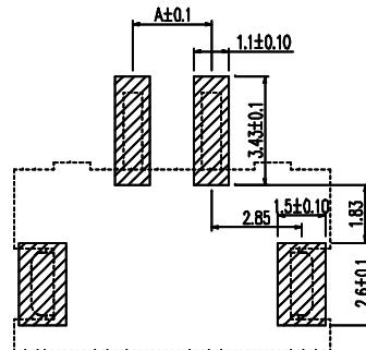
印制线路板
