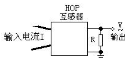
图 1: 输出并联小于 100 欧电阻, 输入 10A 时输出对应 0.5V 不饱和。输出=输出 I*R。
